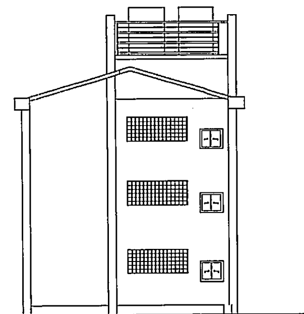
0. FACADE LATÉRALE GAUCHE 1:125
